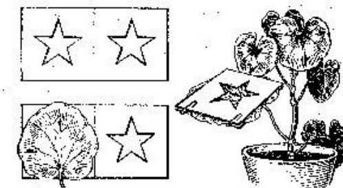
Рис. 30. Получение фигуры Сакса на листе
