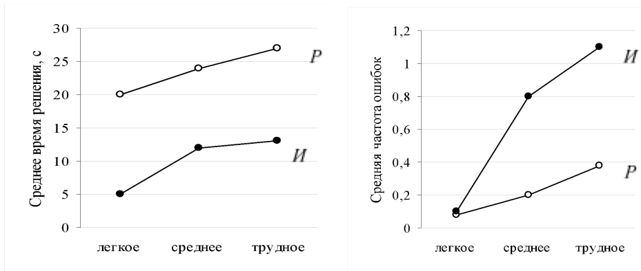
Рис. Решение задач разной степени трудности импульсивными (И) и рефлексивным (Р) подростками
