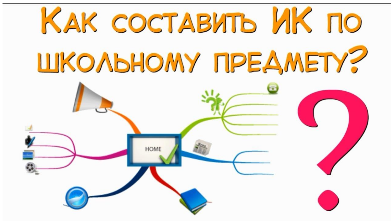
Рис. 1. Схема интеллект-карты
