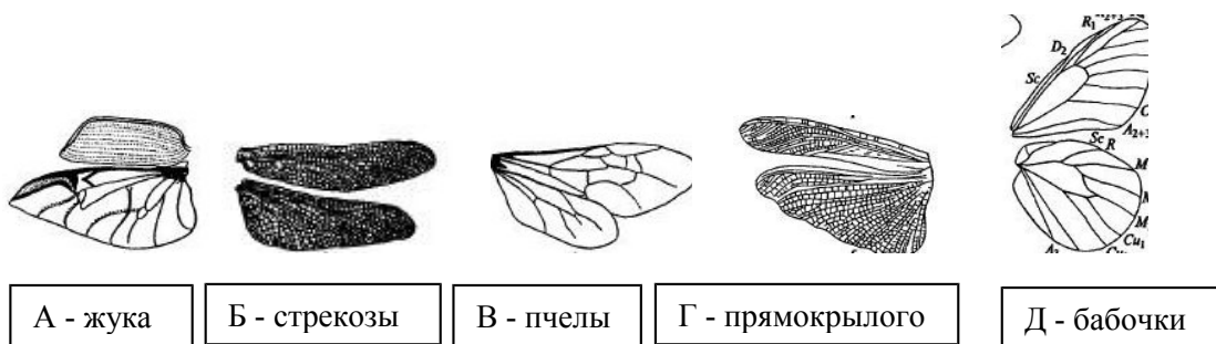
Рис. 10 Крылья насекомых
