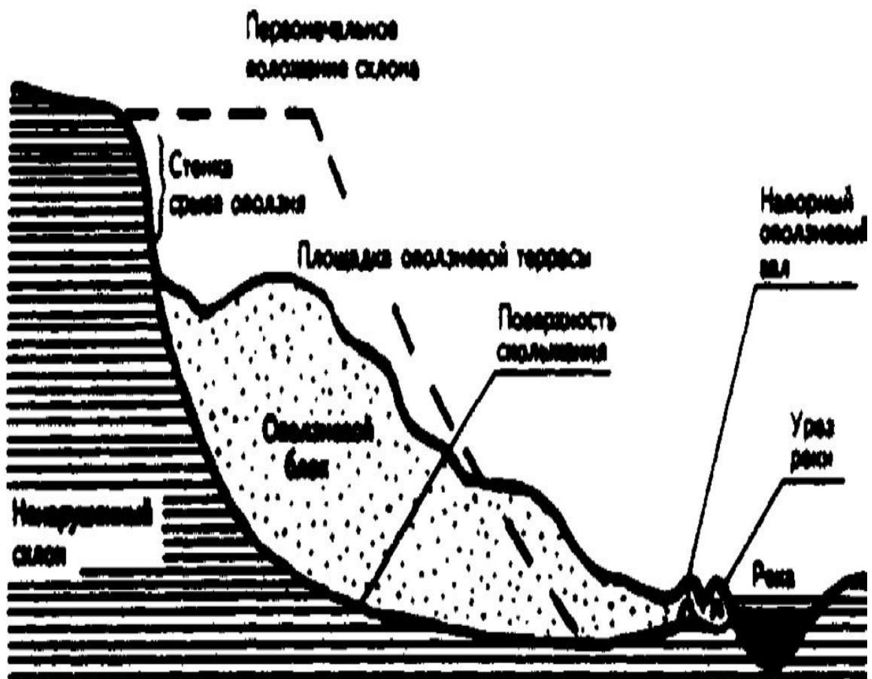
Рис. 4.6. Продольный разрез оползня
