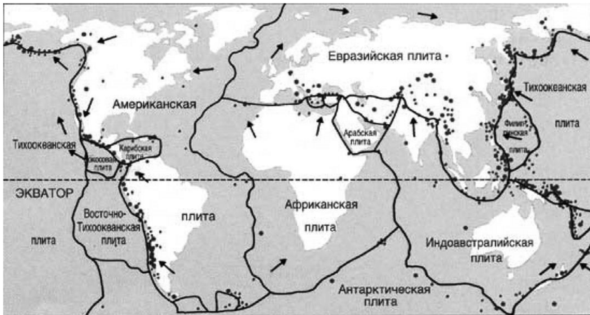
Рис. 3.7 Карта вулканов на Земле
