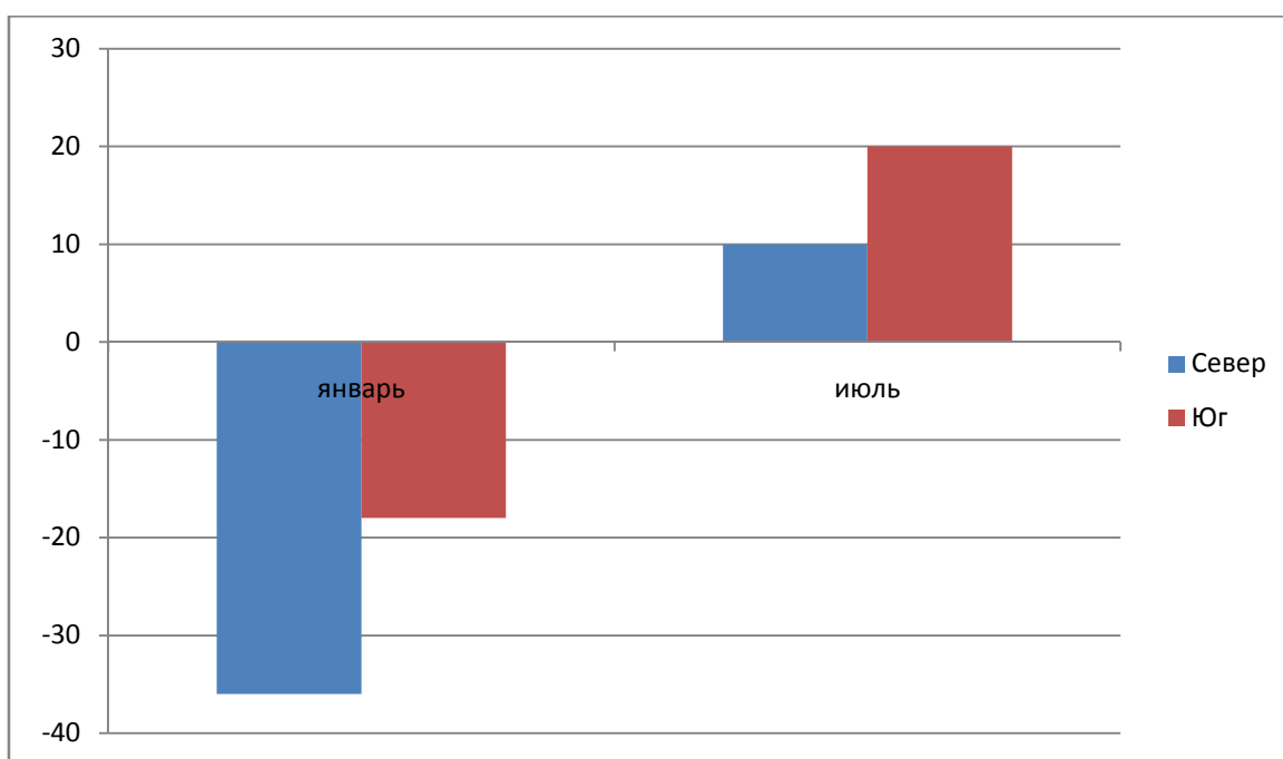
Рис.2 Средняя годовая температура °C на территории Красноярского края.
