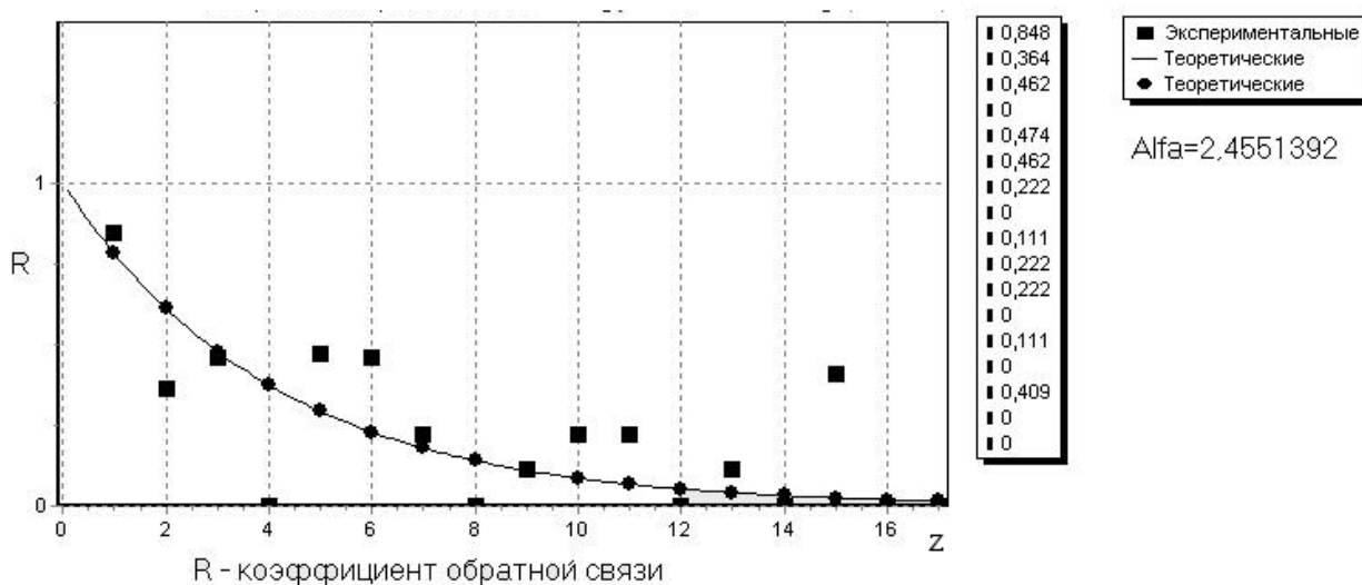
Аппроксимация значений R функцией R = \exp(-\text{alfa} \cdot z)
